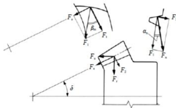
凸齒面為主動時
